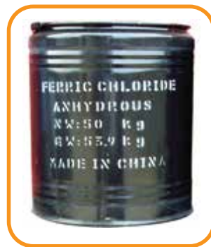
FeCl 3
